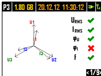
Fig. 5. Pantalla 1 con el gráfico y los indicadores de corrección de conexión.
