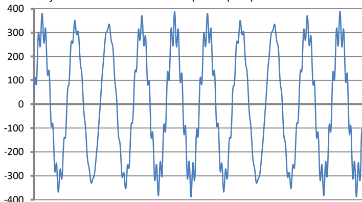
Fig. 47. El efecto de interacción de noveno armónico (450 Hz, 10% Unom) e interarmónico 460 Hz (10% Unom). El cambio visible de envolturas de tensión con una frecuencia de 10 Hz puede causar el parpadeo de la luz (Unom = 230 V RMS, 50 Hz).
