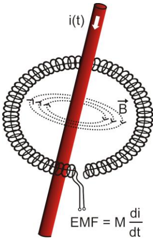
Fig. 45. Bobina de Rogowski
